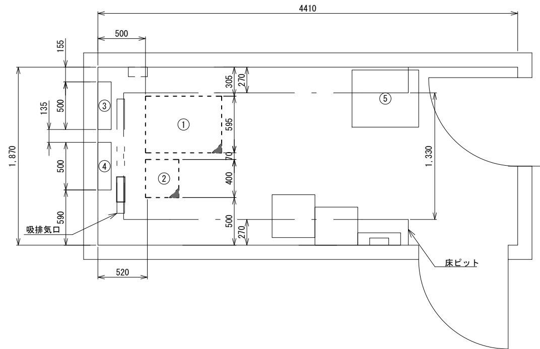
3F防災無線室 平面図 (S=1/20)
