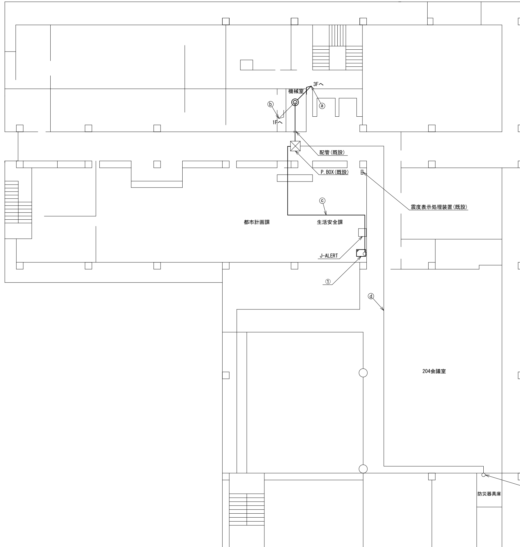
2F平面図 (S=1/100)
