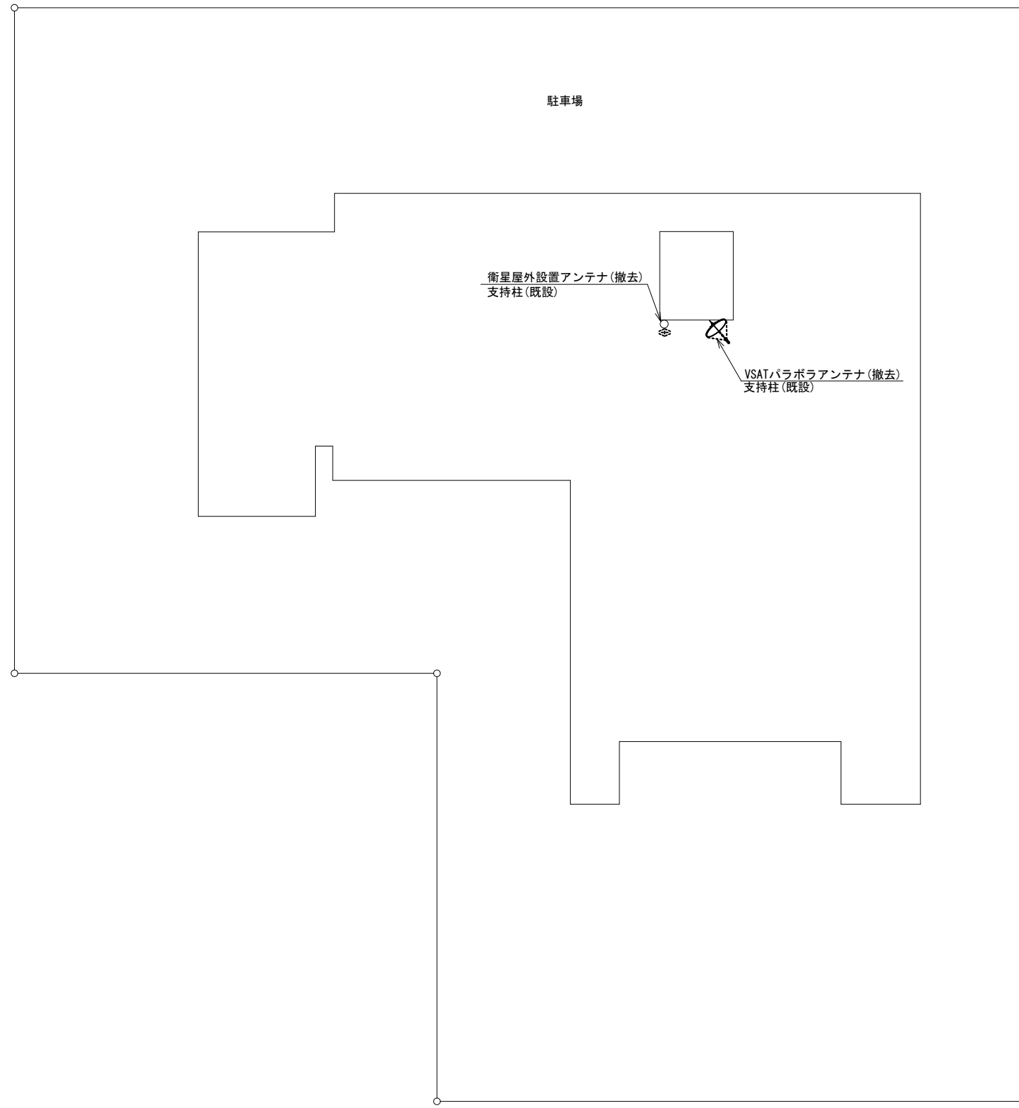
平面図 (S=1/200)
