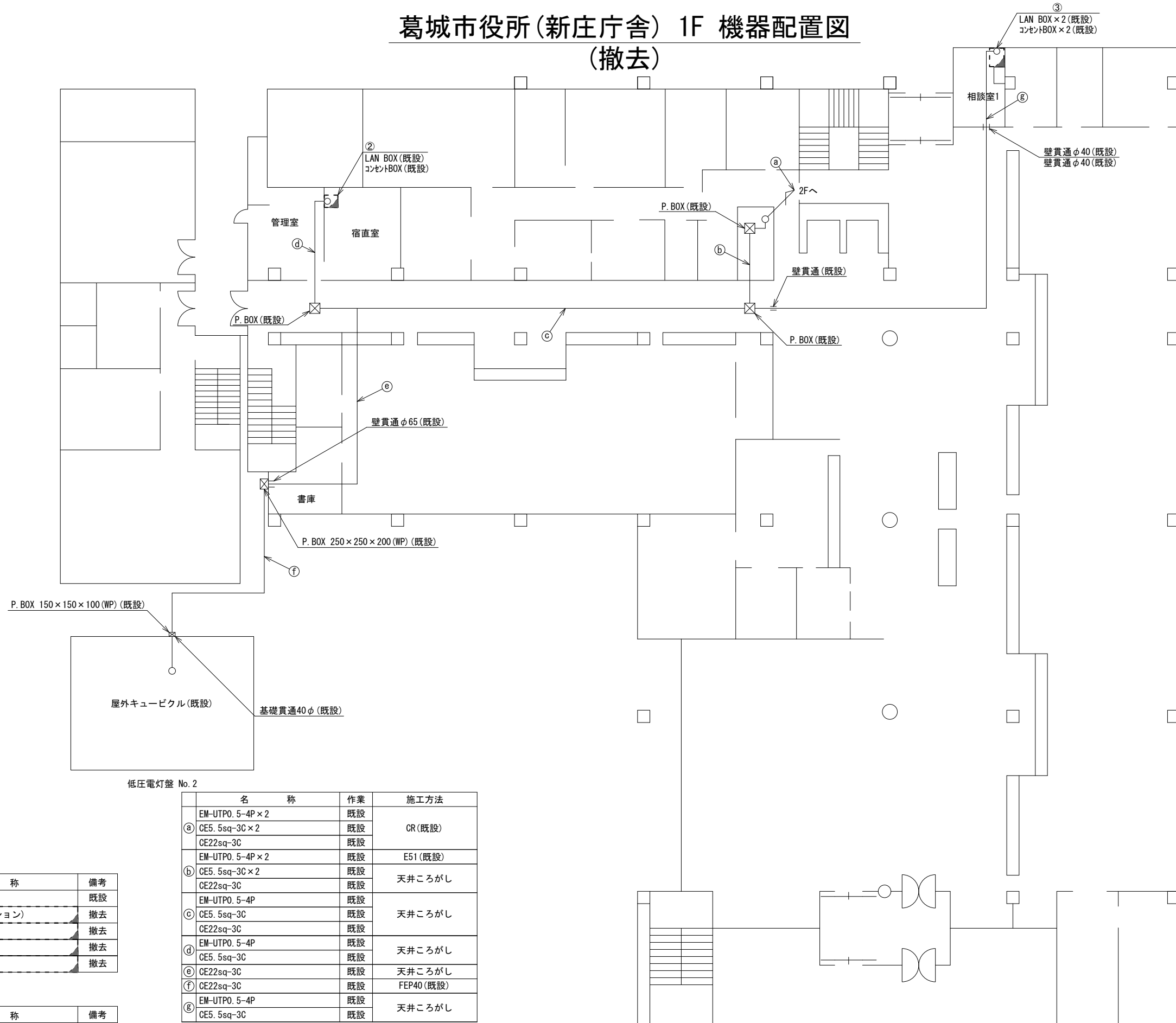
1F平面図(S=1/100)
