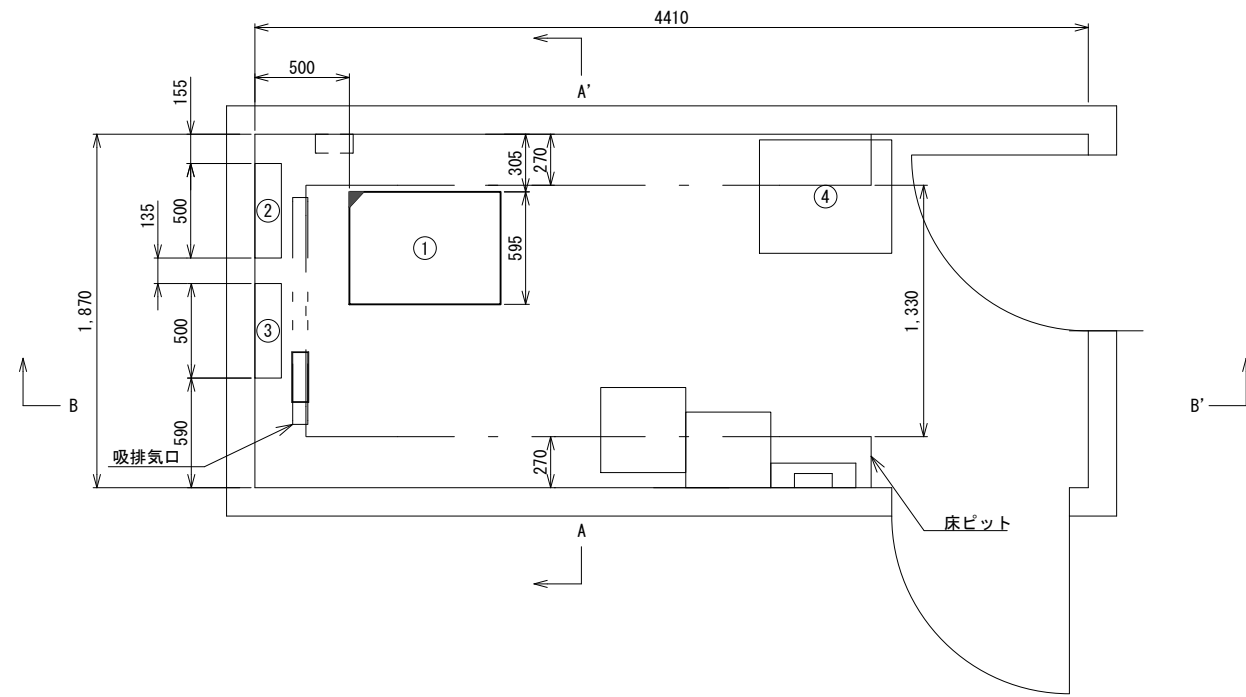
3F防災無線室 平面図 (S=1/20)
